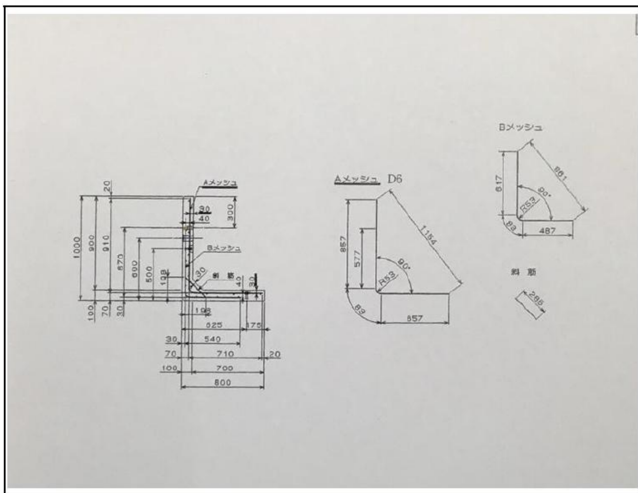
配筋図
