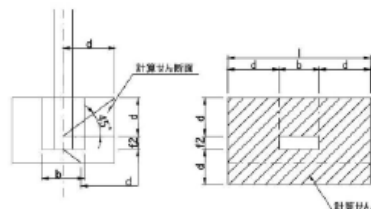
計算せん断面積
