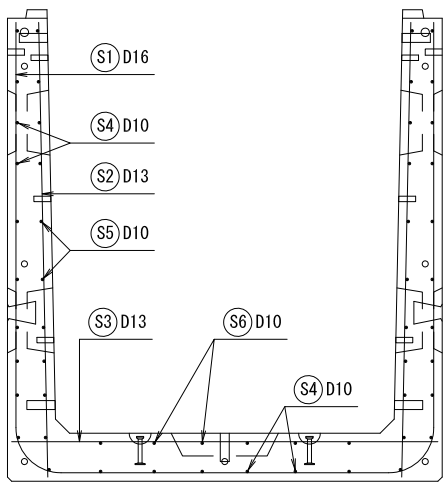
底版 外側 内側
