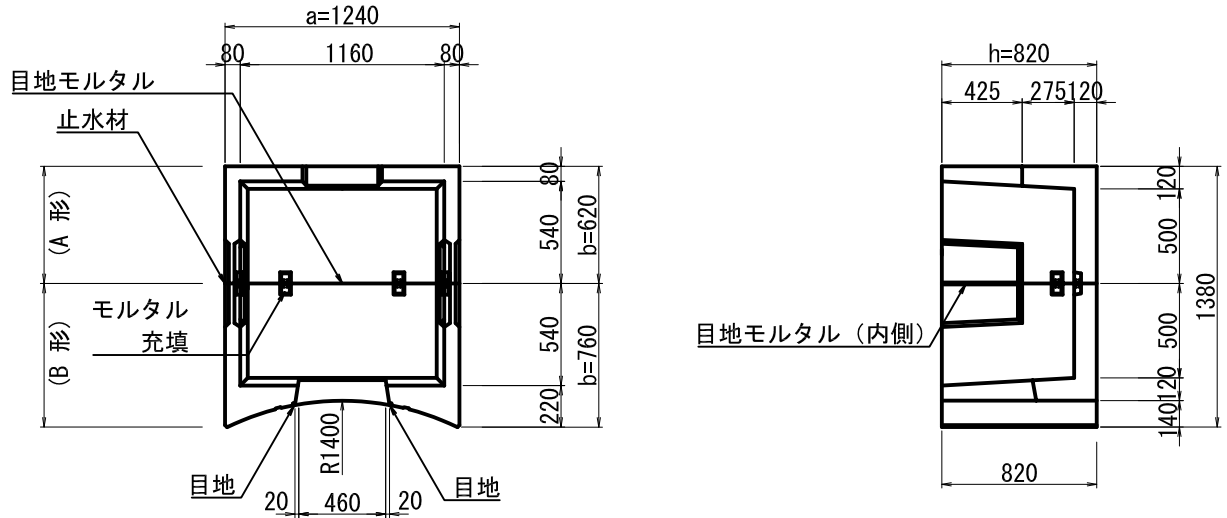
円形落差工用集水桝
